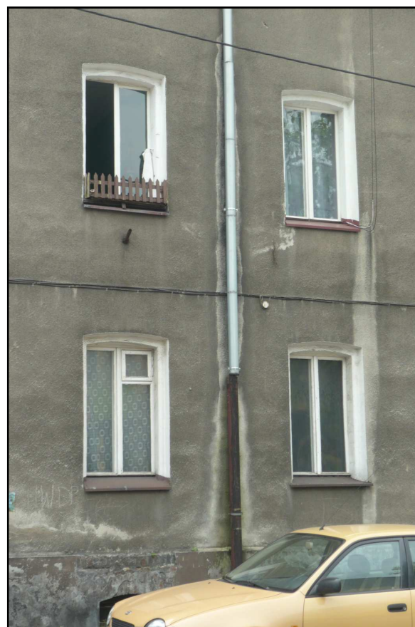
Fot. 15, Fot. 16 Budynek przy ul. Dąbrówki 8. Korozja elementów stalowych, brak ciągłości rury spustowej.
